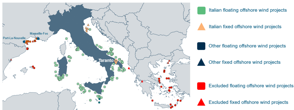
Figura 35 Progetti eolici offshore fissi e galleggianti nel Mar Mediterraneo.
