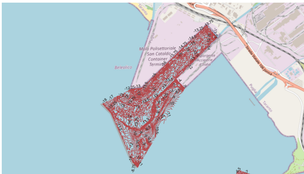
Figura 24 Batimetriche nell'area del Molo Polisettoriale
