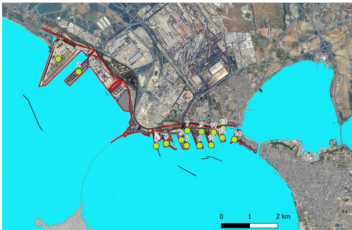
Figura 23 Layout di inquadramento funzionale del porto di Taranto.
