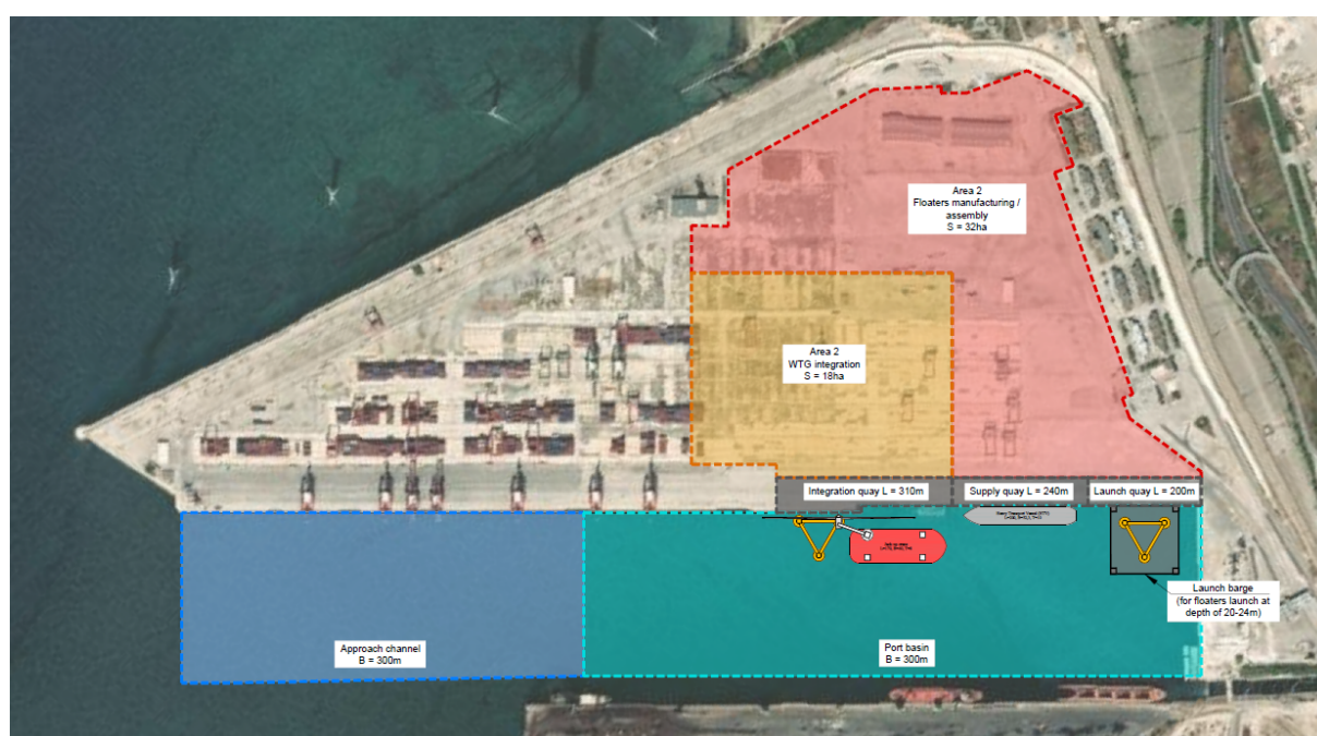
Figura 49 Opzione 1A – Layout preliminare di alto livello al Molo Polisettoriale, Molo 6.
