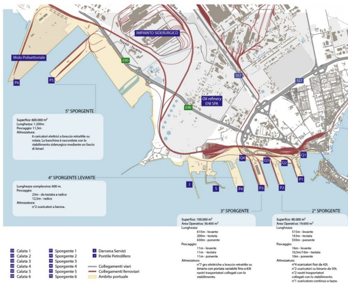
Figura 32 Layout portuale con dotazione ferroviaria del porto.
