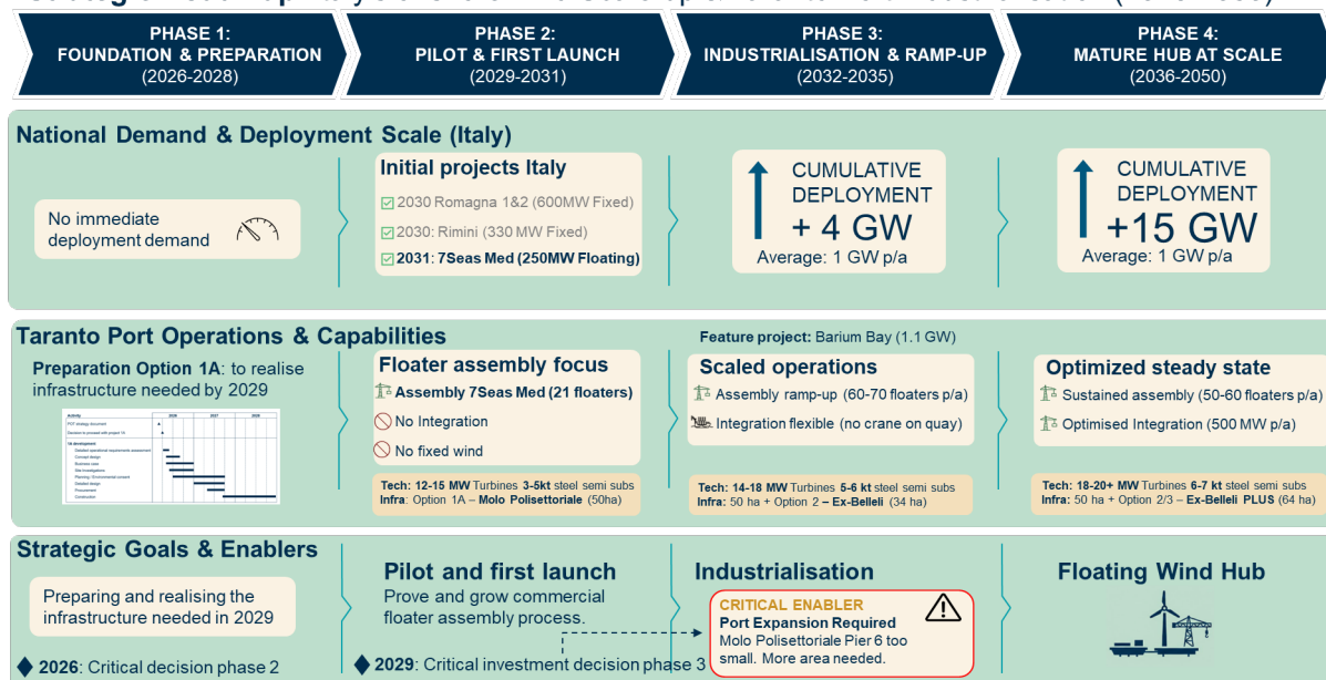
Figura 51 Roadmap strategica per lo sviluppo del Taranto Offshore Wind Hub.
