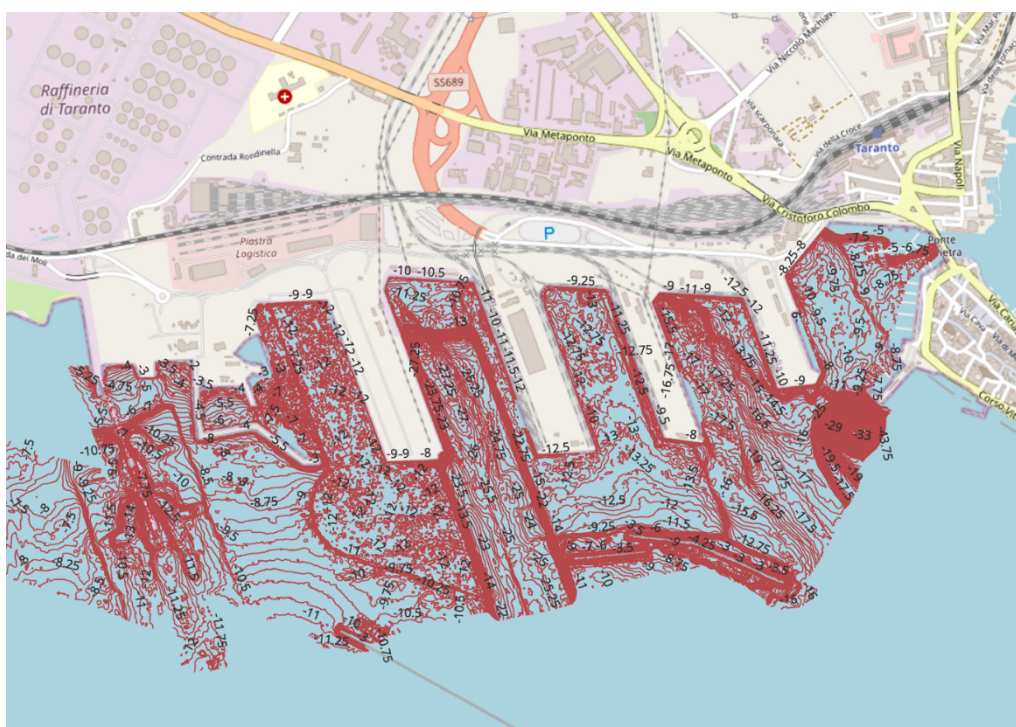
Figura 25 Batimetriche delle calate. Rilievi 2022.
