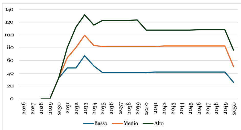
Figura 37 Domanda di aree portuali (ha) per il FOW nei diversi scenari analizzati.
